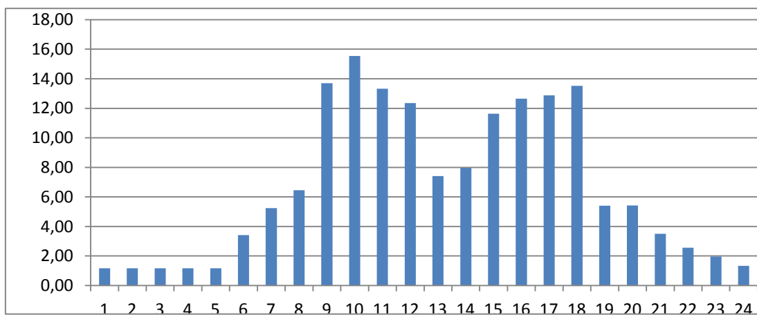
Рис. График распределения расходов д.Евграфовка по часам суток.
