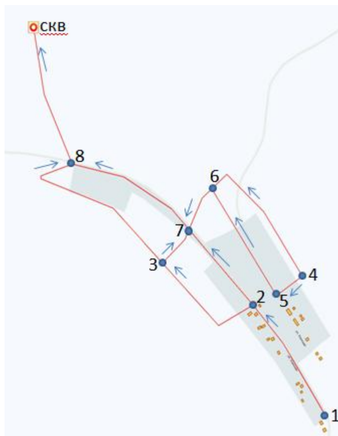
Рис. Разбивка сетей водоснабжения д.Казанка на участки для определения узловых расходов
