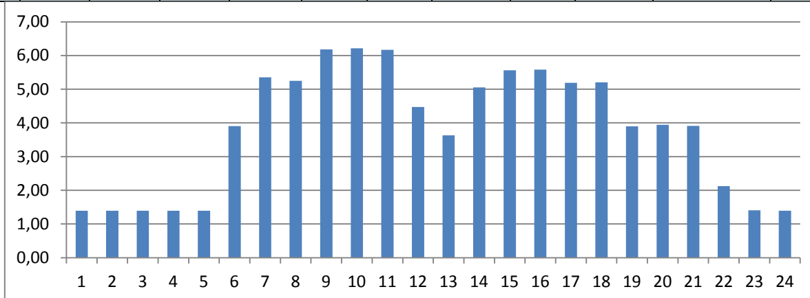
Рис. График распределения расходов с.Покровка по часам суток.
