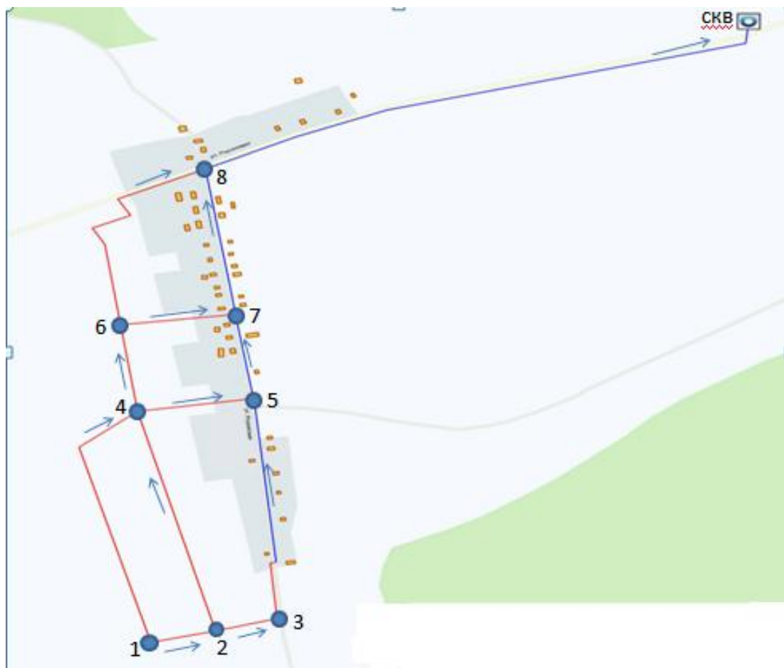
Рис. Разбивка сетей водоснабжения д.Сологубовка на участки для определения узловых расходов
