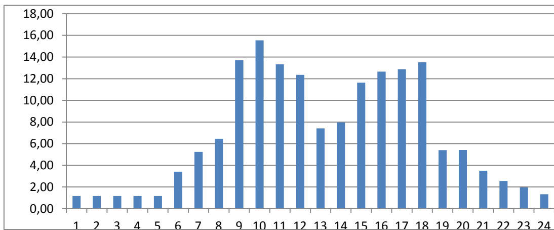
Рис. График распределения расходов д.Дачная по часам суток.
