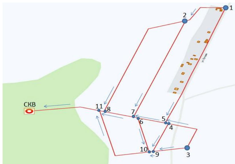
Рис. Разбивка сетей водоснабжения д.Евграфовка на участки для определения узловых расходов
