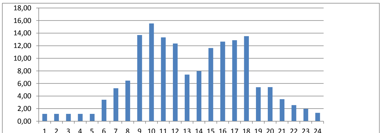
Рис. График распределения расходов д.Казанка по часам суток.
