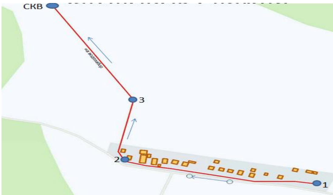
Рис. Разбивка сетей водоснабжения д.Дачная на участки для определения узловых расходов
