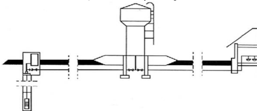
Рис. Схема водоснабжения населенного пункта при заборе воды из подземных источников.
